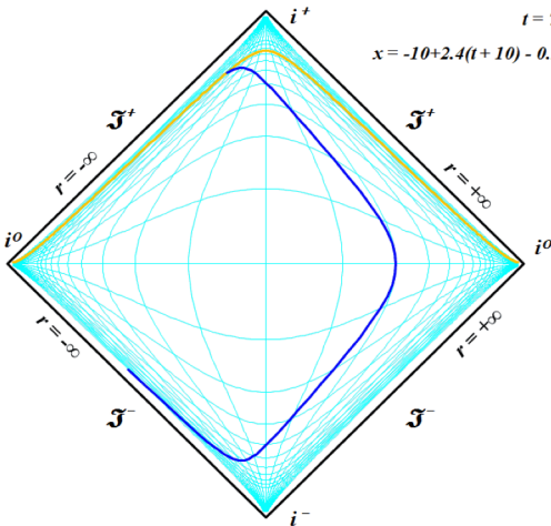
Рис.8.4. Полная диаграмма Пенроуза для всего пространства-времени. На диаграмме в качестве примера изображена мировая линия, описываемая уравнением справа сверху диаграммы [38].
