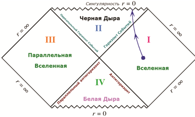
Рис.8.8 Диаграмма Пенроуза для Черной дыры [28]. Диаграмма соответствует традиционному изображению диаграммы шварцшильдвской Черной дыры.
