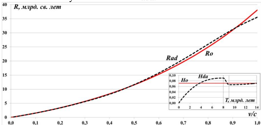
Рис.11.18. При замедленно-ускоренном расширении Вселенной с параметром H_{da} дальние сверхновые видны более тусклыми, а сверхдальние – более яркими. Подбором наугад параметра H_{da} удалось получить вид диаграммы Хаббла, схожий с диаграммой для ускоренного расширения Вселенной.
