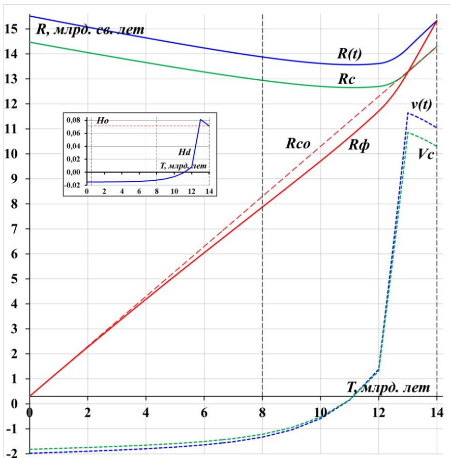
Рис.11.23. Графики движения самой дальней видимой сверхновой в условной, замедляющейся Вселенной с параметром H_d , расширение которой началось буквально вчера.
