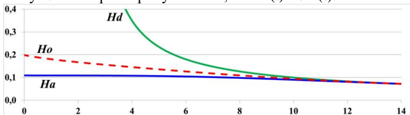
Рис.11.4. Наблюдаемые параметры Хаббла в трёх разных Вселенных, полученные из наблюдаемых диаграмм Хаббла.
