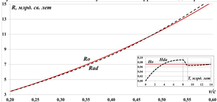
Рис.11.19. Увеличенный фрагмент диаграммы для замедленно-ускоренного расширения Вселенной с параметром H_{da} .
