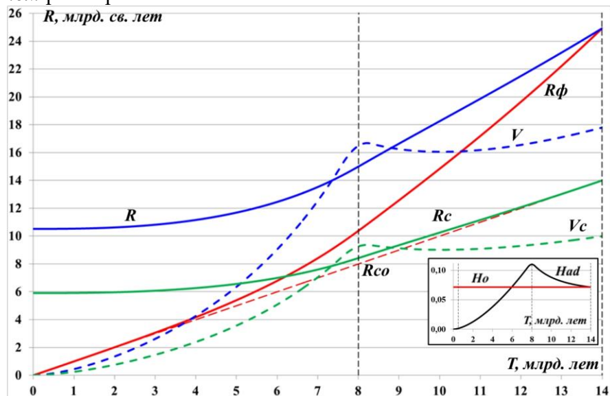
Рис.11.17. Полный набор графиков движения самой дальней видимой сверхновой во Вселенной с параметром H_{ad} – ускоренно-замедленная Вселенная или в принятой терминологии – Вселенная, расширяющаяся замедленно.
