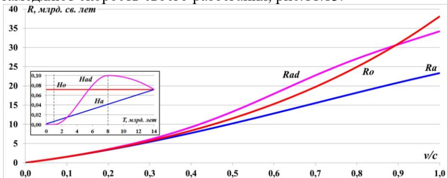
Рис.11.13. Только при ускоренно-замедленном расширении Вселенной H_{da} дальние сверхновые видны более тусклыми, а сверхдальние – более яркими, чем при стандартном расширении Вселенной с неизменным параметром Хаббла H_0 .
