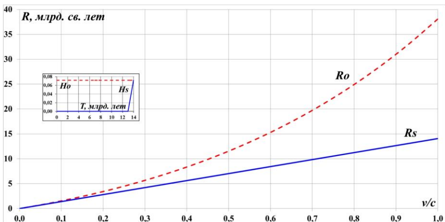
Рис.11.24. Наблюдаемые диаграммы Хаббла для условных Вселенных с параметрами H_0 и H_s .
