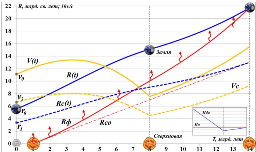
Рис.11.9. Обоснование графиков движения действительного "источника" фотонов. Графики движения сверхновой во Вселенной, расширяющейся с параметром Хаббла H_{da} .
