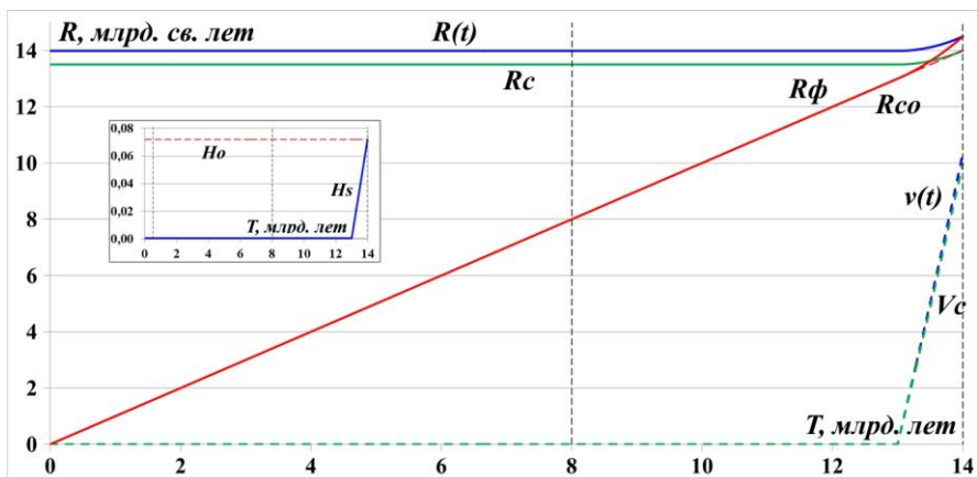
Рис.11.25. Графики движения самой дальней наблюдаемой сверхновой во Вселенной с параметром H_s . Основную часть времени Вселенная стационарна и лишь в последний миллиард лет скачкообразно начала расширение. Параметр Хаббла H_s по наблюдениям будет выглядеть при этом как неизменный и равный современному параметру H_0 в нашей Вселенной.
