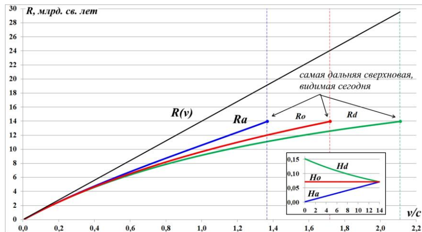
Рис.11.2. Наблюдаемые диаграммы Хаббла для Вселенных с параметрами H_0 , H_d и H_a , соответственно – стандартная (равномерная), замедленная и ускоренная. R_o , R_d , R_a – наблюдаемые диаграммы Хаббла для этих Вселенных, соответственно. Действительная диаграмма Хаббла для всех трёх Вселенных – R(v) .
