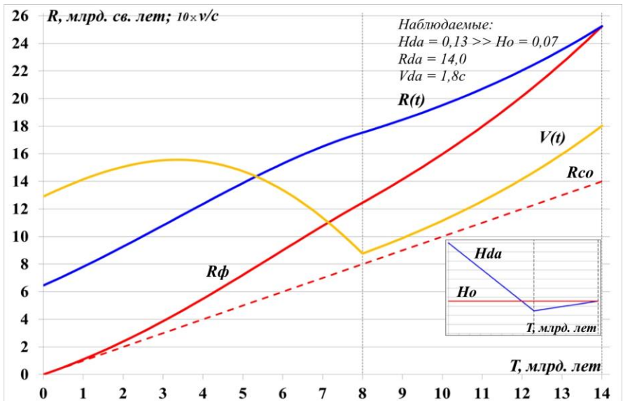
Рис.11.7. Графики движения самой дальней наблюдаемой сверхновой и света от неё в Вселенной, ускоренно расширяющейся с параметром Хаббла H_{da} .
