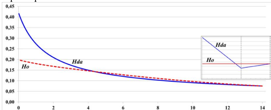
Рис.11.6. Зависимости от времени наблюдаемых параметров Хаббла в ускоренной и равномерной Вселенной. На врезке – исходные параметры Хаббла. Как видим, наблюдаемые параметры отличаются от исходных, причём они монотонно убывают, что выглядит как замедленное расширение Вселенной.
