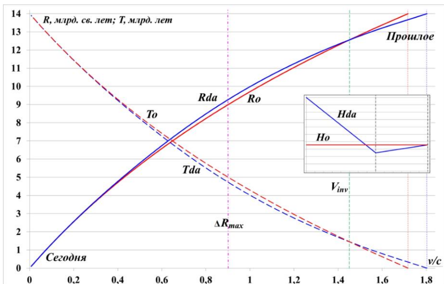
Рис.11.5. Наблюдаемые диаграммы Хаббла для Вселенной с H_0 и Вселенной с H_{da} , расширяющейся сначала замедленно, затем ускоренно. Графики соответствующих параметров Хаббла приведены на врезке. В ускоренной Вселенной дальние сверхновые видны более тусклыми, они дальше.
