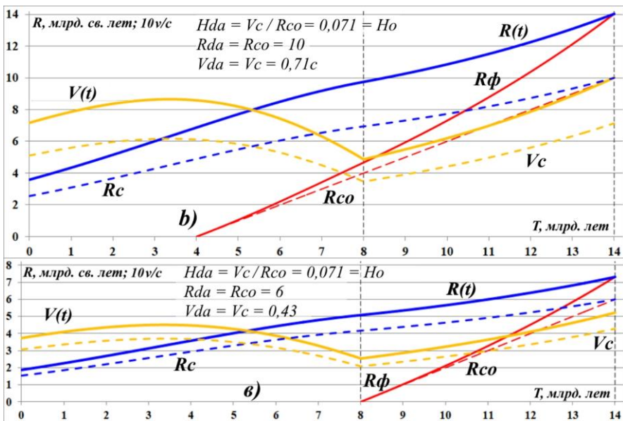
Рис.11.8. Графики движения Rc и Vc действительного "источника" фотонов для разных сверхновых.
