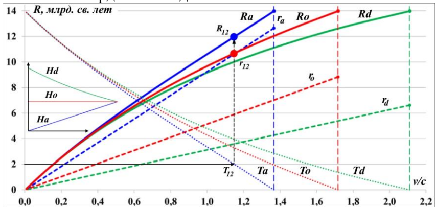
Рис. 11.3. Наблюдаемые диаграммы Хаббла, графики времени и начальных удалённостей сверхновых для Вселенных с параметрами H_0 , H_d и H_a .
