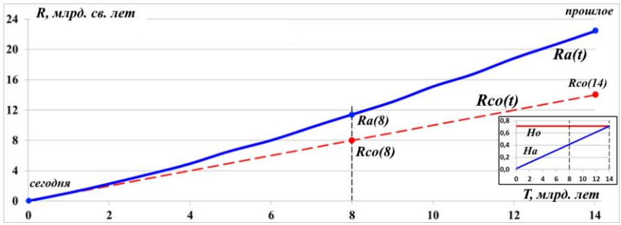
Рис.11.11. График значений действительной, реально наблюдаемой удалённости Ra(t) самой дальней сверхновой, находившейся в момент вспышки на разных удалёностях от Земли с учётом времени в пути света от вспышки. Пример для сверхновой, вспыхнувшей 8 млрд. лет назад: Ra(8) – наблюдаемая дальность, Rc(8) – путь, пройденный фотонами.
